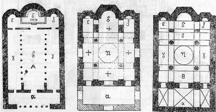
Σχέδια Βυζαντινῆς ἐκκλησίας.
