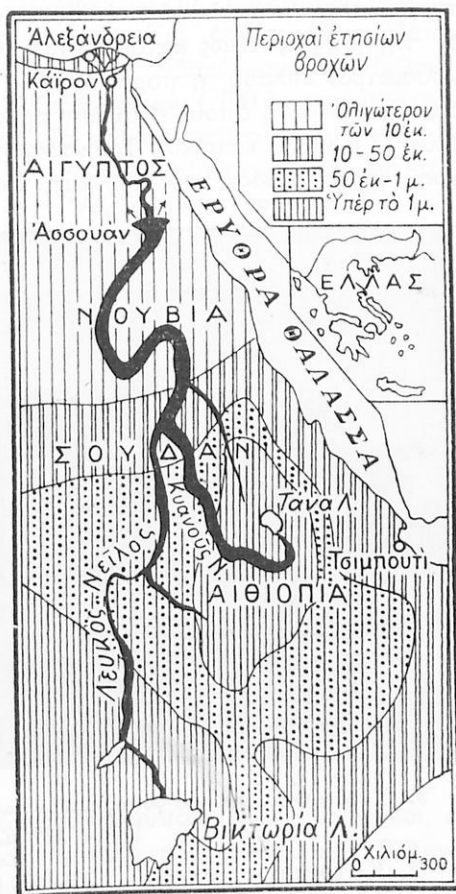
56. Ἡ ἐτησίως κατερχομένη ποσότης τῶν ὑδάτων τοῦ Νεῖλου μέχρι τοῦ Ἀσσουάν καὶ ἡ διατηρουμένη κατὰ τὸν ὑπόλοιπον ροὺν αὐτοῦ.
