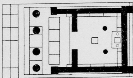
Σχ. 2. Ναὸς πρόστυλος
