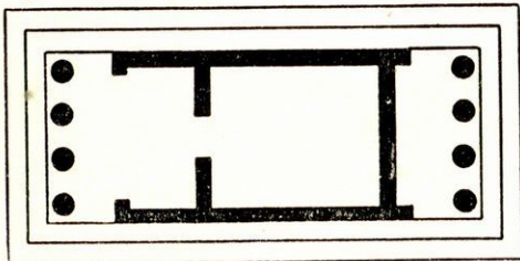
Σχ. 3. Ναὸς ἀμφιπρόστυλος
